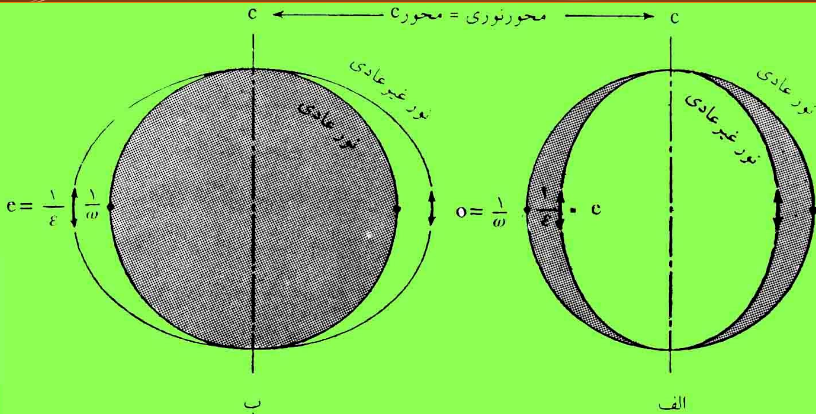
شکل ۲-۳. نمایش مقاطع سطح موجها در بلورهای یک محوری مثبت و یک محوری منفی. الف) بلور یک محوری مثبت، ب) بلور یک محوری منفی.
