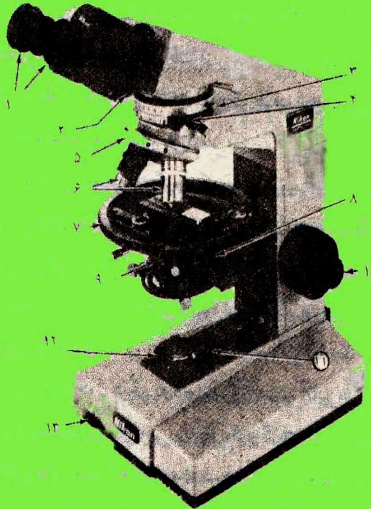
شکل ۳-۴. نمایش قسمتهای یک میکروسکوپ پلاریزان
