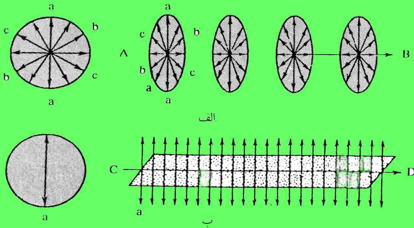
شکل ۱-۵. الف) نور معمولی با تقارن محوری درجه بینهایت، ب) نور پلاریزه با تقارن صفحه‌ای.
